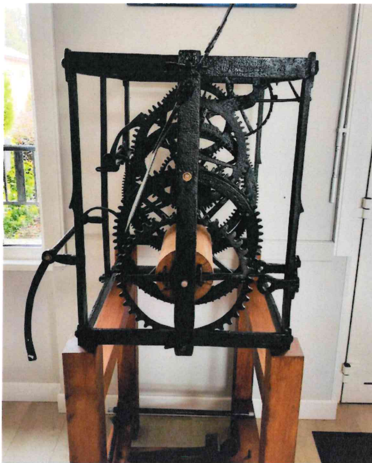
Mécanisme d'horloge-cage (cl. Ville de Nalliers)
