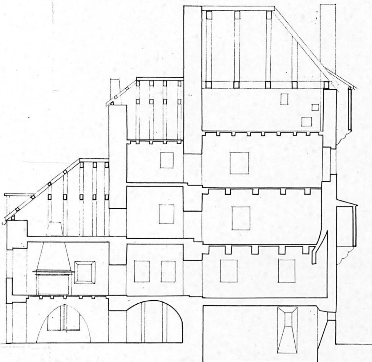
COUPE VV'
