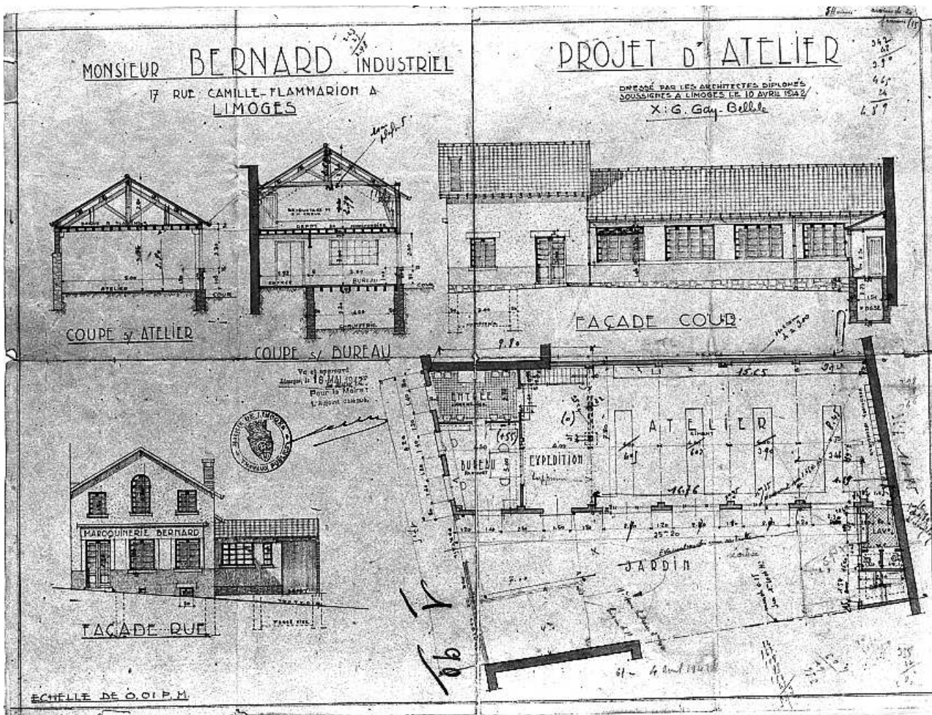
Doc.1 « Monsieur Bernard Industriel – 17 rue Camille-Flammarion – Limoges – 03870008V Dressé par... le 10 avril 1942 ». Plan, tirage mis en couleur, 1 : 100, 54 x 40,4 cm, 10/04/1942. AC Limoges : Série 1 O 216 - Permis n°179 (90) – 4 mai 1942.
